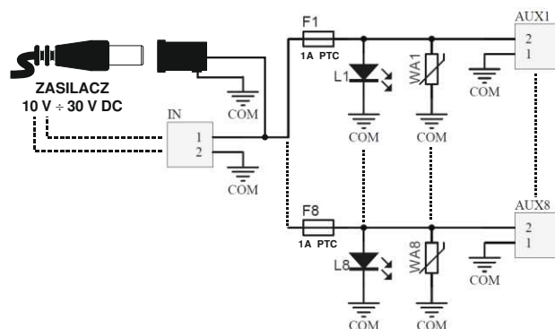
Rys.2. Schemat elektryczny.
